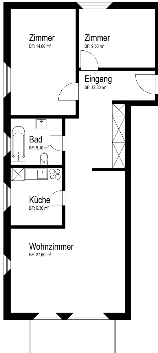
Wohnung 4
